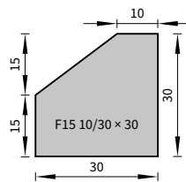
Platte boordstenen
