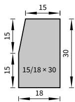
Hoge boordstenen
